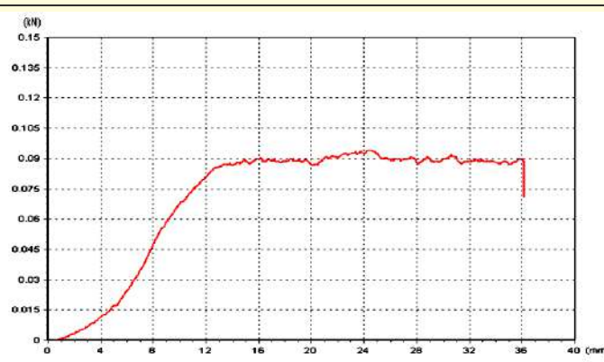
Courbe de la force de désolidarisation sur un déplacement de plusieurs cm. On peut remarquer que lorsque la qualité de vulcanisation est bonne (comme dans cet essai), la force de désolidarisation est constante, avec une force moyenne de désolidarisation de 9DaN pour une largeur de bande de 100mm.
