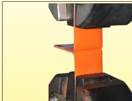
Echantillon après vulcanisation, avant le test de désolidarisation
